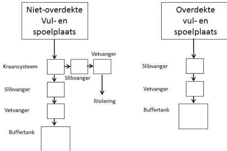
Figuur 3: diagram voor de opbouw van een vul- en spoelplaats
