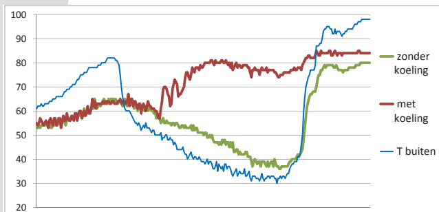
Effect van natte koeling op de RV (5/06/2015 - dag 31)
