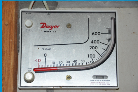
De onderdruk in de stal is bepalend voor de luchtverdeling in de stal.
