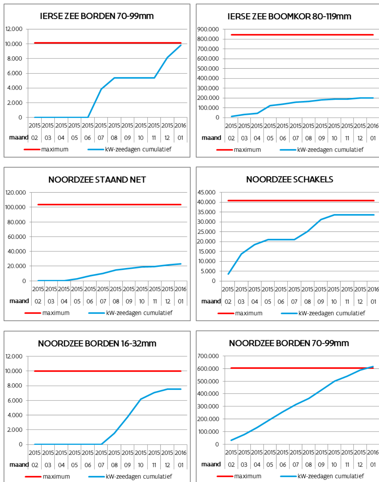
Grafiek 27: Cumulatieve visserij-inspanning in de kabeljauwherstelgebieden beheerperiode 2015
